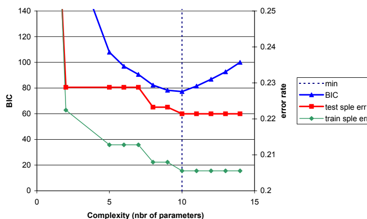
FIG. 1 – BIC sur échantillon d'apprentissage et taux d'erreur.
